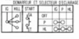
RACCORDEMENT DU CONTACTEUR D'ALLUMAGE, DEMARREUR ET SELECTEUR DECLAIRAGE
